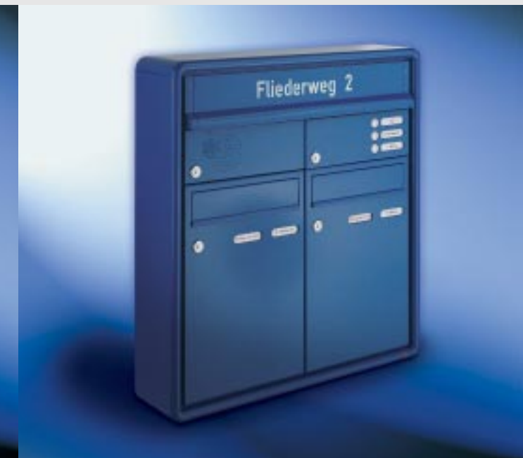
Abb. 53/3 Kastenformat 300 x 440 x 145 mm, mit RS50 und RS4, Beleuchtungskasten, 2. Namensschild mit Aufschrift „Werbung, nein danke!“, ALU-Verkleidungsprofil RS 2000.
