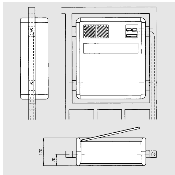
Einbaubeispiel: Durchwurf-Zaunbriefkasten.
