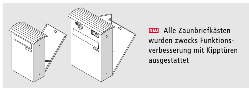
Bestell-Nr. 17-0-17057 Kastenformat 436 x 581 x 185 mm, mit RS50 und RS4, JUMBO-Zaunbriefkasten aus Edelstahl V4A mit CONVEX®-Dach.
